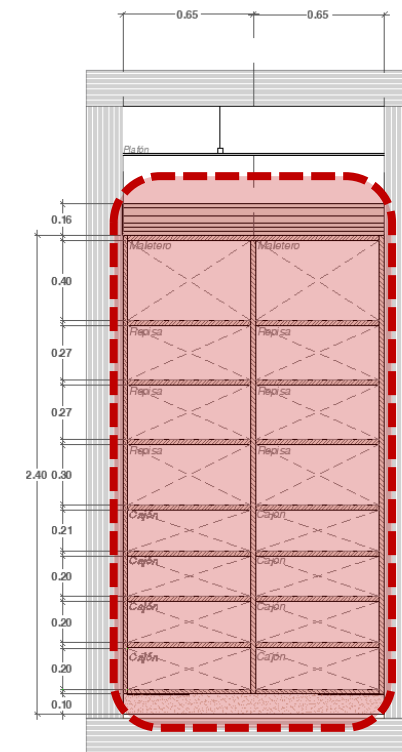
3. Linen closet
